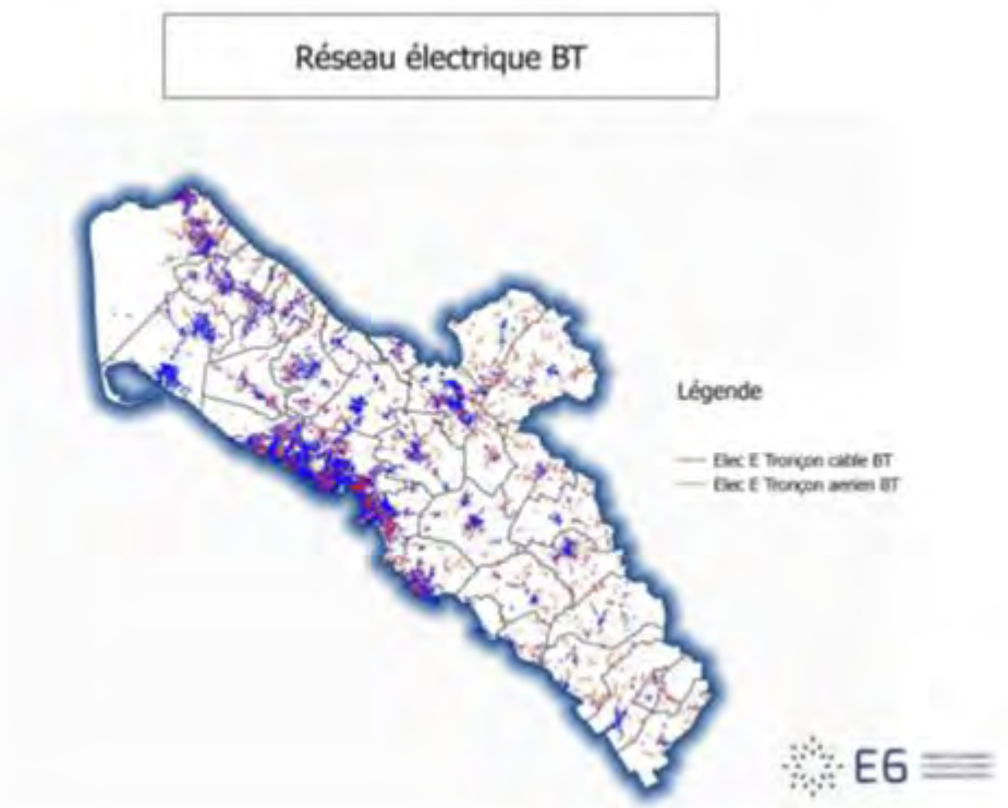
FIGURE 52 : RESEAU BASSE TENSION, 2017 ; SOURCE : DIAGNOSTIC DES RESEAUX DE TRANSPORTS ET DE DISTRIBUTION, E6 CONSULTING 2018
