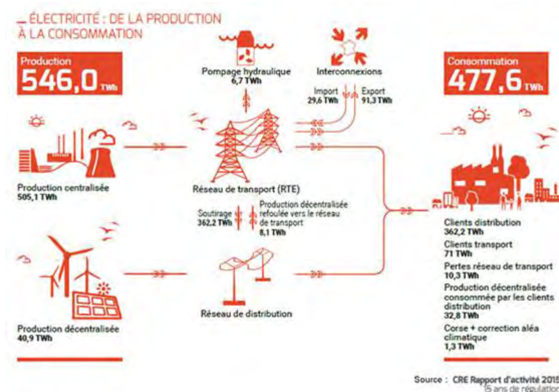
FIGURE 50 : SCHEMA DE L'ELECTRICITE, DE LA PRODUCTION A LA SOURCE ; SOURCE : DIAGNOSTIC DES RESEAUX DE TRANSPORTS ET DE DISTRIBUTION, E6 CONSULTING 2018
